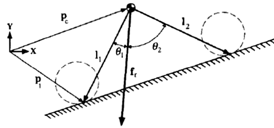
شکل ۳ شماتیک از معیار پایداری نیرو-زاویه در حالت دوبعدی [۲۲]
