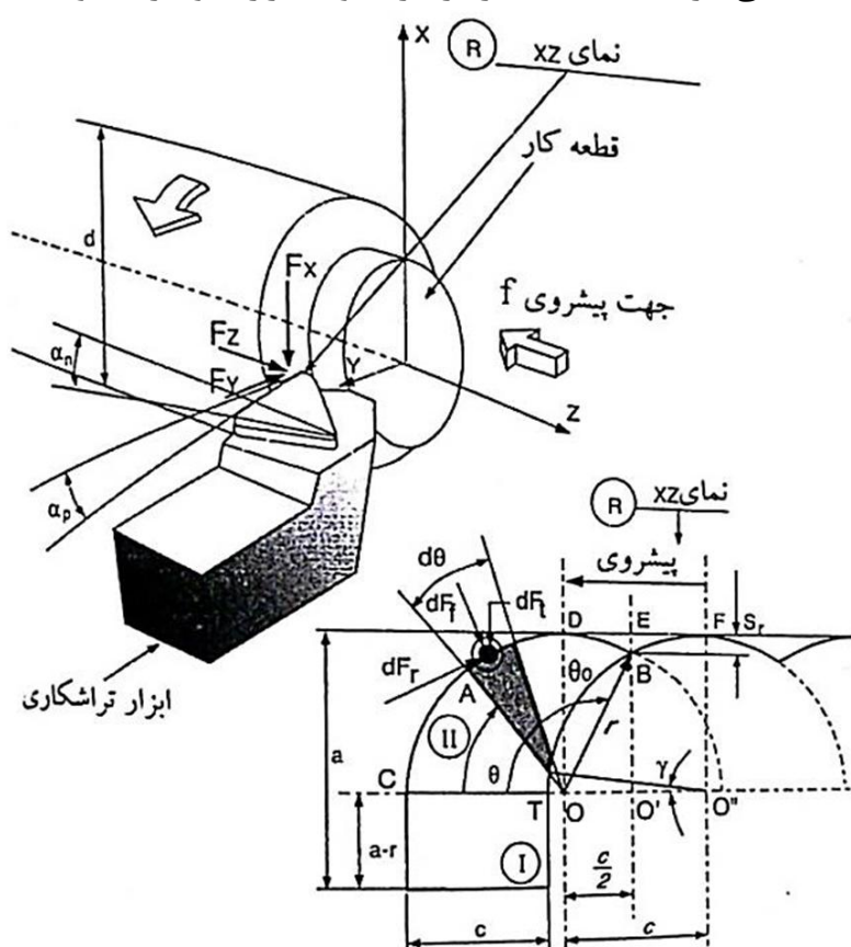
شکل 1 شماتیک فرآیند تراش کاری به وسیله اینسرت با نوک شعاع دار [20]
