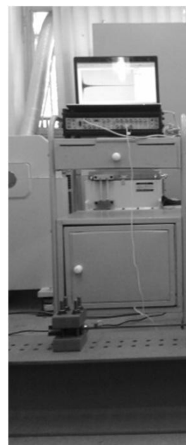
شکل 9 استخراج پاسخ ارتعاش تیر فولادی با شتاب‌سنج پیزوالکتریک Type4507 شرکت B&K و دستگاه داده‌برداری چهار کاناله Type 3109
