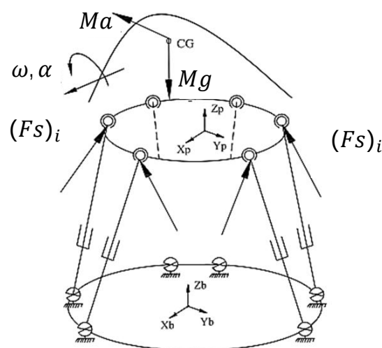
شکل 3 آنالیز دینامیک، ہم بازوی، ربات
