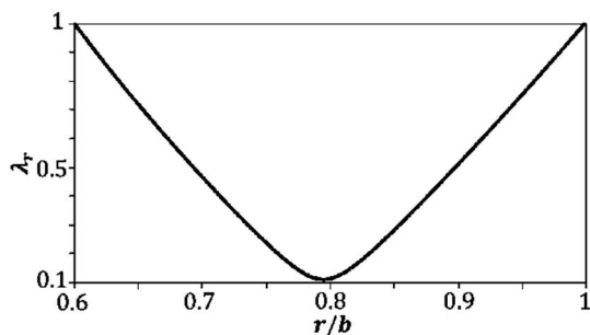
Fig. 6 Yield variable changes throughout thickness under internal pressure 5 MPa and thermal difference 91°C for parameters m_1=-3 , m_2=0.5 , m_3=-0.5 and m_4=0.5 شکل 6 تغییرات متغیر تسلیم در طول ضخامت برای فشار داخلی 5 MPa و اختلاف دمای 91 °C برای مشخصات m_1=-3 , m_2=0.5 , m_3=-0.5 و m_4=0.5 اگر آن تحت تنها بارگذاری فشار داخلی قرار داده شود و فشار تا حد رخ دادن تسلیم بالا برود، با توجه به تغییرات پارامترها به نتایج جدول 3 می‌توان رسید.
