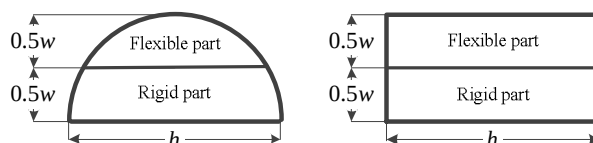
Fig. 12 Cross-section of partial flexible circular and rectangular struts شکل 12 سطح مقطع میله‌های دو-تکه دایره‌ای و مستطیلی
