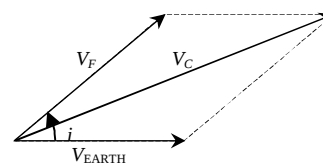
Fig. 3 Required orbital velocity with consider Earth's rotation شکل 3 سرعت مورد نیاز مداری با در نظر گرفتن چرخش زمین
