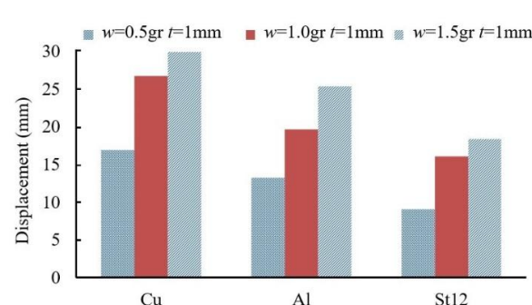
Fig. 18 Maximum experimental deflection of circular plate's with 1mm thickness by different explosive charges in different materials شکل 18 حداکثر تغییر شکل تجربی مرکز ورق دایروی با ضخامت 1 میلی‌متر برای خرج‌های انفجاری مختلف در جنس‌های متفاوت
