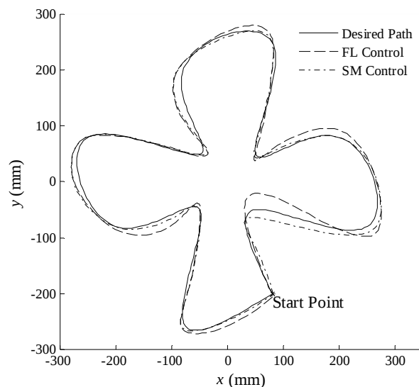
Fig. 4 Desired and actual paths
