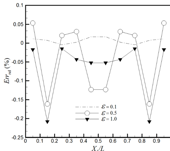
Fig. 3 The relative errors for estimating the total heat flux over the design surface for three different values of gray wall emissivity, \tau = 1 شکل 3 نمودار توزیع درصد خطای نسبی شار حرارتی روی سطح طراحی برای سه مقدار مختلف ضریب صدور دیواره‌های خاکستری محفظه، \tau = 1
