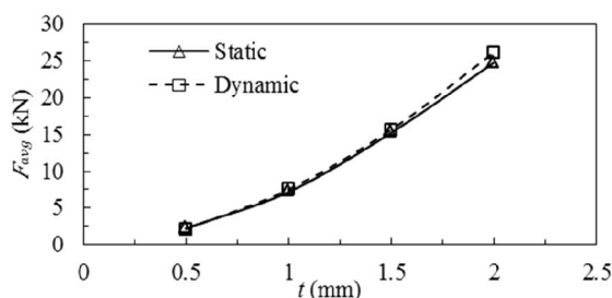
Fig. 5 Variations of mean crushing force vs thicknesses of square tube شکل 5 تغییرات نیروی متوسط لپیدگی برای ضخامت‌های مختلف لوله مربعی
