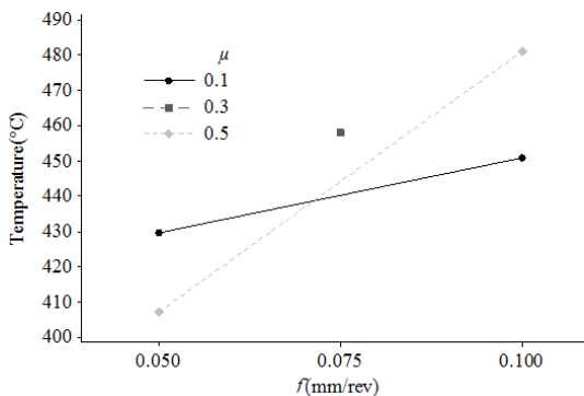
Fig. 9 Interaction plot of friction coefficient and feedrate on temperature of the cutting edge شکل 9 اثر متقابل ضریب اصطکاک و پیشروی بر دمای لبه برنده ابزار
