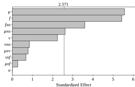
Fig. 11 Pareto chart for DOS
