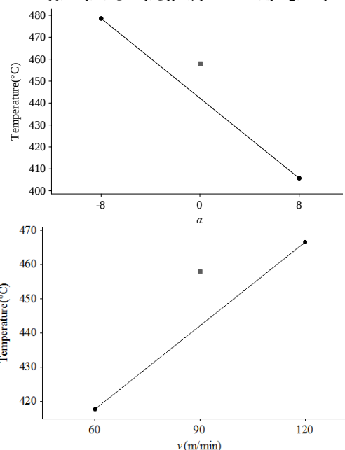
Fig. 10 Main effects of cutting speed and rake angle on temperature of the cutting edge شکل 10 نمودار اثرات اصلی سرعت برشی و زاویه براده بر دمای لبه برنده ابزار
