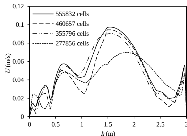
Fig. 8 Velocity on the line (x = 1.5, x = 1.5) in terms of height شکل 8 توزیع سرعت روی خط (x = 1.5, z = 1.5) برحسب ارتفاع
