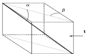
Fig. 3 Inclined cable subjected to wind with slope \alpha and yaw angle \beta شکل 3 کابل شیب‌دار با شیب \alpha و زاویه انحراف \beta در معرض باد
