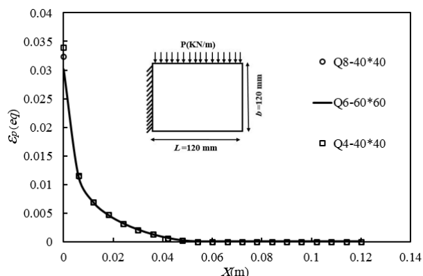
Fig. 12 Equivalent plastic strain through the plate length for Q4, Q6 and Q8 elements at y=120\text{mm} and 0 < x < 120\text{ mm} شکل 12 نمودار کرنش معادل پلاستیک در راستای طول صفحه برای المان‌های Q4، Q6 و Q8 در y=120\text{mm} و 0 < x < 120\text{ mm}
