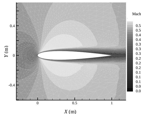
Fig. 14 Mach contour of viscous laminar subsonic flow in order of N=3 شکل 14 کانتور عدد ماخ برای جریان زیرصوت آرام لزج در مرتبه N=3
