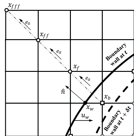
Fig. 4 Schematic of grid nodes for the illustration of moving boundary شکل 4 شماتیکی از نقاط گرهی برای تشریح مرز متحرک
