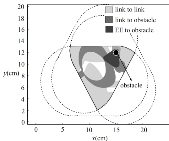
Fig. 7 Collision-free workspace of the 3-PRR parallel robot for \theta=30^\circ . شکل 7 فضای کاری عاری از تداخل مکانیکی ربات موازی 3-PRR برای جهت‌گیری \theta=30^\circ
