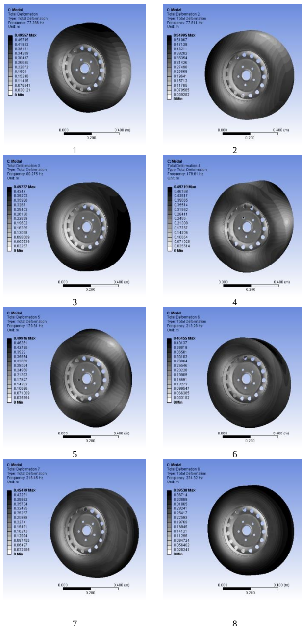
Fig. 20 The first eight natural frequencies and modes of tire and rim model شکل 20 مدهای هشت فرکانس طبیعی اول مدل تایر و رینگ
