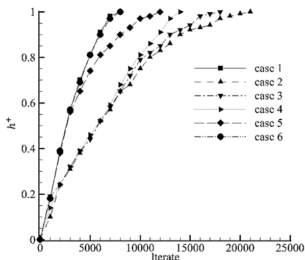
Fig. 14 Penetration of fluid in porous medium for different states شکل 14 نفوذ سیال به درون محیط متخلخل در حالات مختلف
