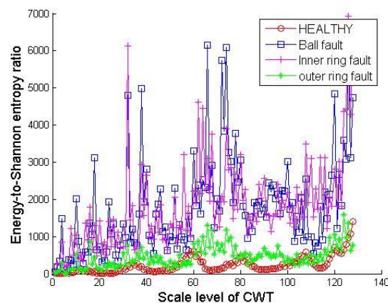
Fig. 4 Optimum Scales
