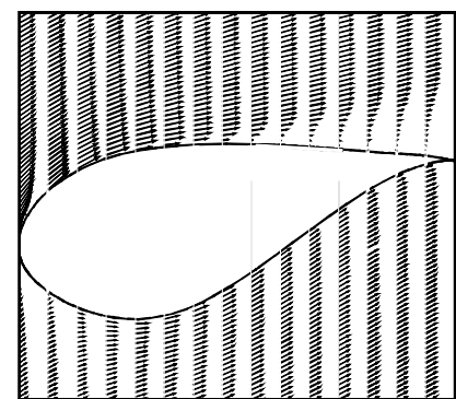
(الف) عملگر غیرفعال
