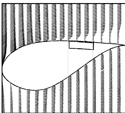
(ج) عملگر فعال حالت 2
