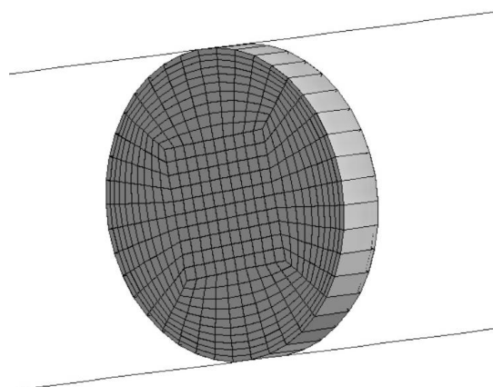
Fig. 2 Used mesh
