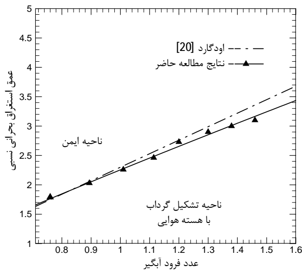
شکل 12 عمق استغراق بحرانی نسبی بر حسب عدد فرود آبنگبر برای آبنگبر منفرد افقی
