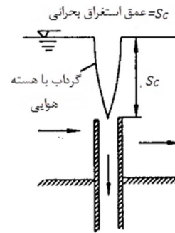
شکل 1 نمایش عمق استغراق بحرانی آبیگری
