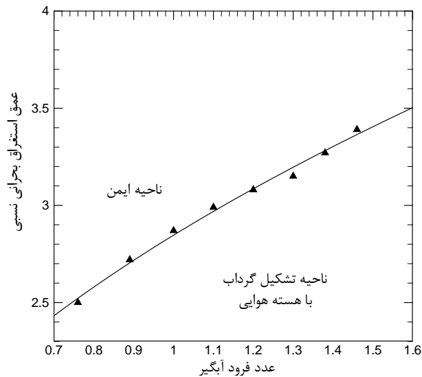
شکل 11 نتایج بدست آمده برای عمق استغراق بحرانی نسبی در برابر عدد فرود آبنگبر برای آبنگبر مایل
