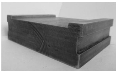
Fig. 3 The flattened die
