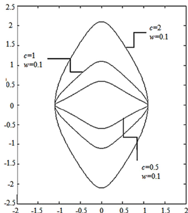
شکل 3 تأثیر پارامتر c بر هندسه گشودگی
