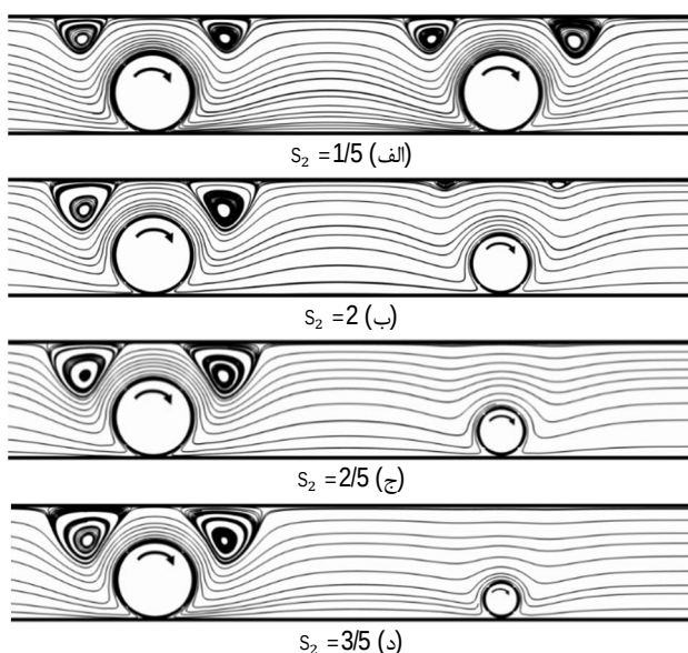
شکل 6 خطوط جریان درون ریزمجرا برای S_2 های مختلف و S_1 = 1/5 در حالت \varepsilon_1 = \varepsilon_2 = 0/9 و L = 3
