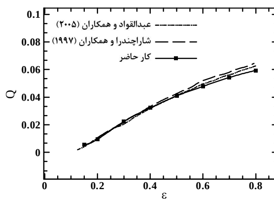
شکل 3 مقایسه نتایج دبی خروجی از میکروپمپی با تک روتور دایروی در کار حاضر با نتایج دیگران
