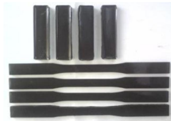
شکل 5 نمونه‌های استفاده شده برای انجام آزمایش‌های مکانیکی نانوکامپوزیت
