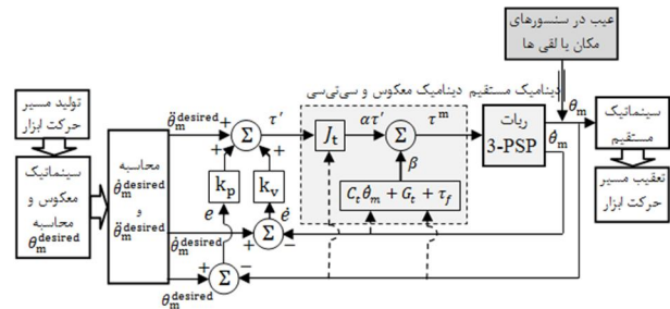
شکل 12 نحوه و مکان اعمال عیب 2 و مدل کنترلی متناظر با آن
