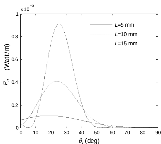
شکل 8 نمودار جریان توان متوسط مود M3 در اتصال چسبی سه لایه آلومینیوم-اپوکسی-آلومینیوم برای یک منبع با ابعاد محدود برحسب پارامترهای ترنسدیوسر تابش زاویه‌ای در فرکانس 0/25MHz
