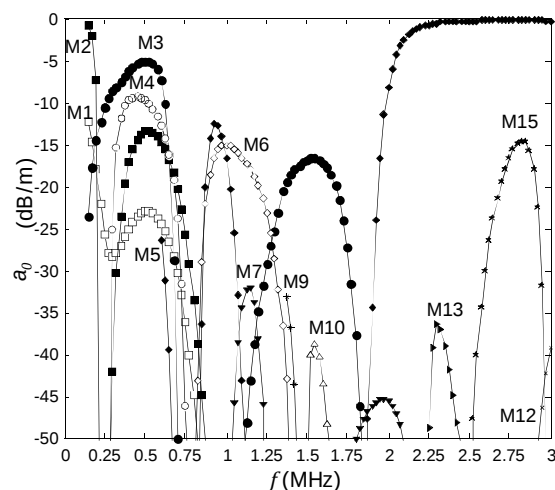
شکل 6 نمودار تجزیه اتلاف برحسب فرکانس برای مودهای مختلف در اتصال چسبی سه لایه آلومینیوم-اپوکسی-آلومینیوم
