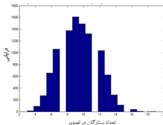
شکل 9 توزیع ستارگان در کره آسمان برای میدان دید 15 درجه و قدر 6 کاتالوگ یکنواخت شده به روش ذرات باردار برحسب فاصله
