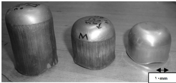
شکل 18 نمونه‌های شکل گرفته در دماهای به ترتیب از راست به چپ: دمای محیط، 150°C، 450°C
