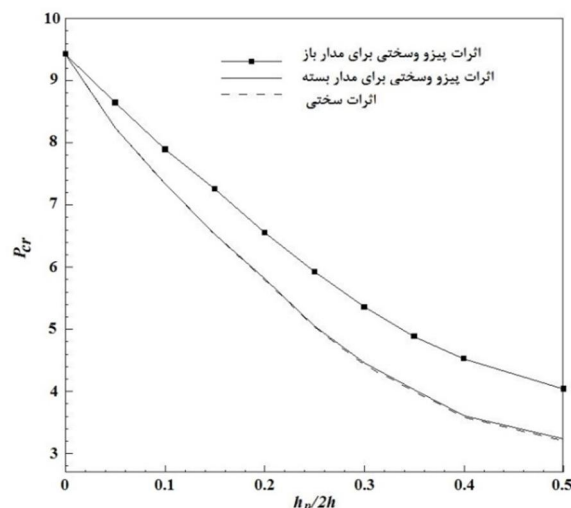
شکل 7 تغییرات بار بحرانی کماتش بی بعد بر حسب نسبت ضخامت‌ها، اثر پیزو برای حالت مدار باز و بسته ( R=1, N=5, a/b=0.5 )
