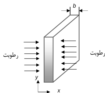
شکل 4 شماتیک نفوذ رطوبت در یک لایه نازک چسب
