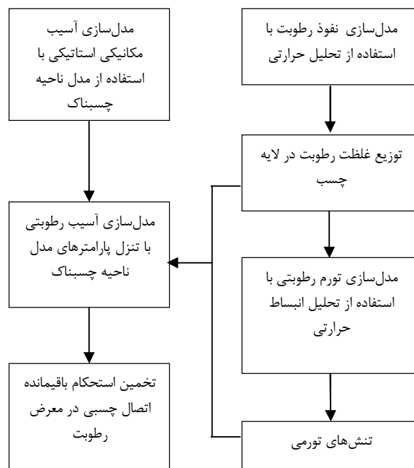
شکل 12 فرایند کامل تخمین استحکام باقیمانده‌ی یک اتصال چسبی در معرض رطوبت با لحاظ تنش‌های تورمی
