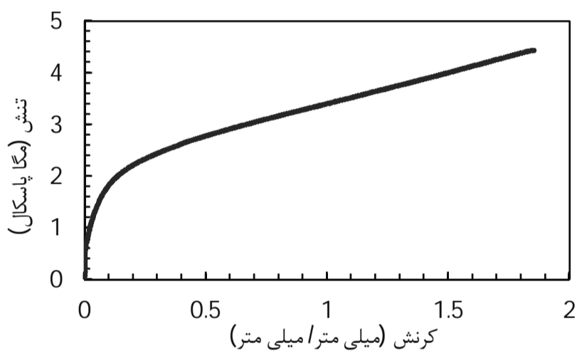
شکل 4 نمودار تنش- کرنش لاستیک
