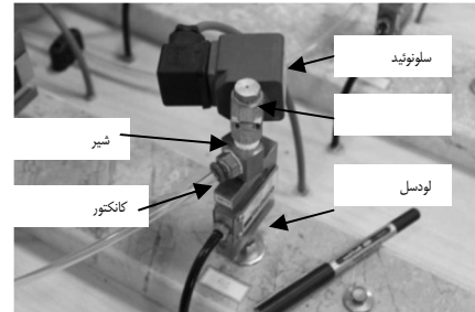
شکل 1- مجموعه تراستر گاز سرد
