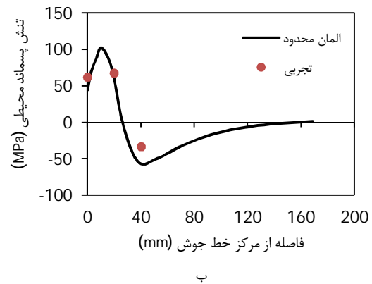
شکل 12 مقایسه تنش‌های پسماند ناشی از المان محدود با نتایج تجربی الف. تنش پسماند محوری ب. تنش پسماند محیطی
