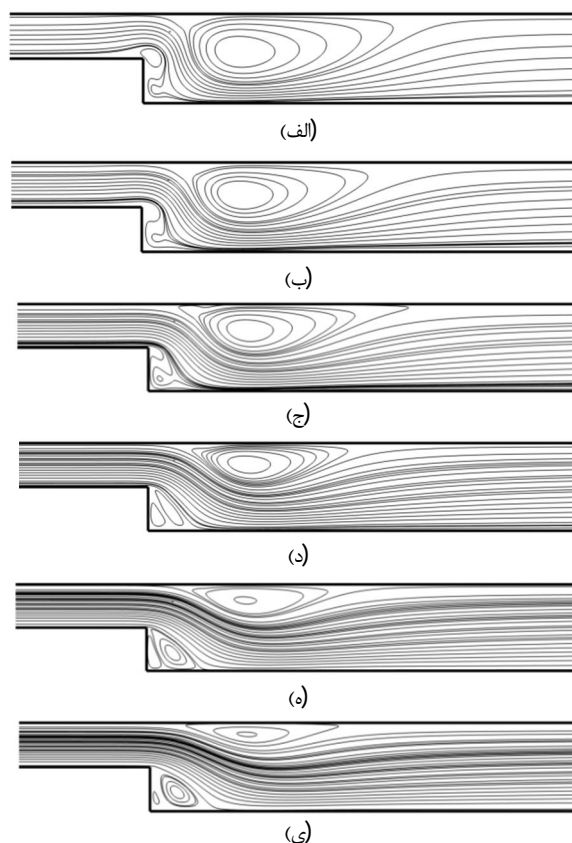
شکل 12 تاثیر عدد رینولدز بر جریان سیال V=18\text{ kV} , \alpha = 45^\circ (الف) \text{Re}=770 (ب) \text{Re}=1050 (ج) \text{Re}=1330 (د) \text{Re}=1610 (ه) \text{Re}=1890 (و) \text{Re}=2170 (ز)
