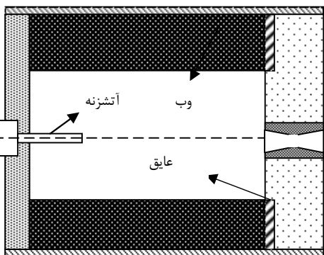
شکل 5 شماتیکی از محل قرارگیری عایق و آتشنزه در موتور
