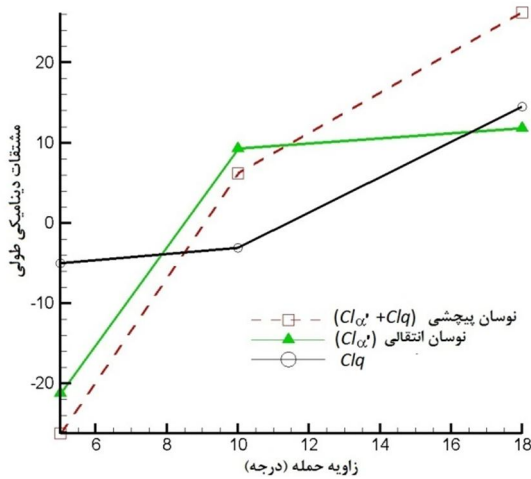
شکل 17 تغییرات مشقتات دینامیکی طولی ضریب برآ با زاویه حمله متوسط، \bar{\alpha}=5^\circ , V=30\text{m/s} , k=0/06
