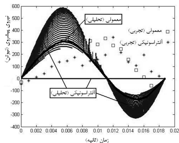
شکل 11 مؤلفه نیروی برشی در جهت پیشروی ( F_y ) تجربی و تحلیلی در فرزکاری معمولی و آلتراسونیکی در آزمایش شماره 2
