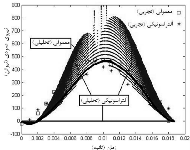
شکل 10 مؤلفه عمودی نیروی برشی ( F_x ) تجربی و تحلیلی در فرزکاری معمولی و آلتراسونیکی در آزمایش شماره 2
