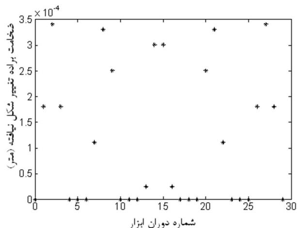
شکل 2 ضخامت براده تغییر شکل نیافته در موقعیت زاویه‌ای \theta=30 در دور گردش متوالی ابزار با شرایط f=21732 Hz و a=5 \mu m، N=500 rpm
