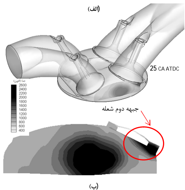
شکل 12 شکل شعله در مسعی اس، عرضی و ب: طولی از سیلندر
