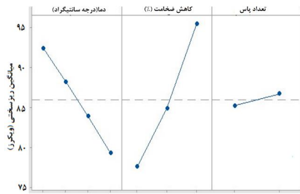
شکل ۱۳) بررسی اثرات اصلی متغیرهای دما، درصد کاهش ضخامت و تعداد پاس بر میانگین ریزسختی
