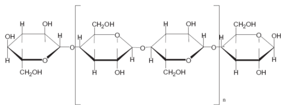
شکل ۲) ساختار شیمیایی سلولز [25]
