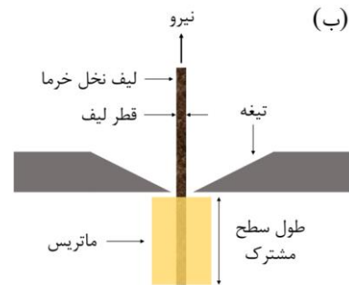
شکل ۵) نمونه و فیکسچر تست Pull-out، (ب) نمای شماتیک تست Pull-out و اجزای مختلف آن
