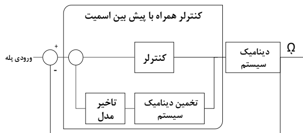
شکل 6 بلوک دیاگرام روش اسمیت
