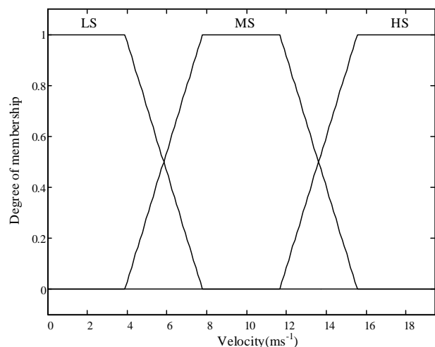
Fig. 6 Membership functions of first input (Instant speed) شکل 6 توابع عضویت ورودی اول (سرعت لحظه کنونی)
