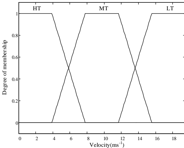
Fig. 7 Membership functions of second input (Traffic intensity) شکل 7 توابع عضویت ورودی دوم (شدت ترافیک)
