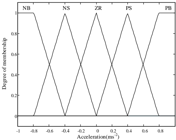
Fig. 8 Membership functions of output (Acceleration) شکل 8 توابع عضویت خروجی (شتاب)
