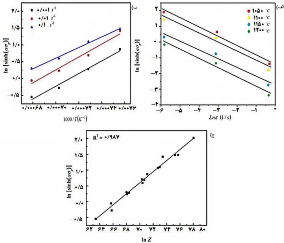
شکل ۳) ارتباط بین الف) \ln[\sinh(\alpha\sigma)] ، \ln \epsilon ، ب) \ln[\sinh(\alpha\sigma)] و 1000/T ، ج) \ln Z و \ln[\sinh(\alpha\sigma)] مورد بررسی در پژوهش حاضر با استفاده از معادله هایپربولیک در 0.0095 = \alpha
