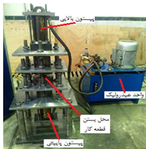
شکل 4 دستگاه پرداختکاری با جریان ساینده
