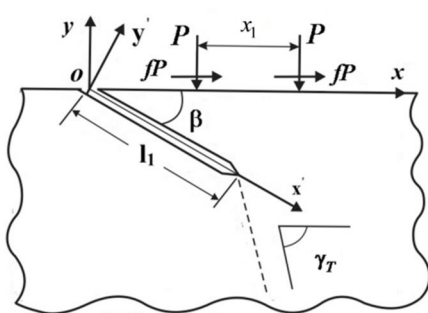
شکل 9 مدل فیزیکی مسئله مورد بررسی همراه با دو بار متمرکز متحرک
