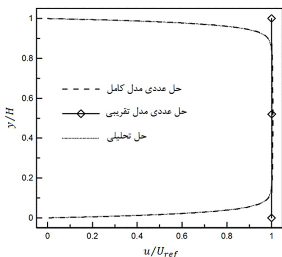
شکل 3 مقایسه تغییرات سرعت درون ریزمجرای همگن به ازای حل عددی مدل کامل، مدل تقریبی هلمهولتز-اسمولوکوفسکی و حل تحلیلی میدان سرعت الکترواسموتیک برای E_{ext} = 14/59 \text{ v/mm} و k = 41 و \zeta^* = 25 \text{ mv}
