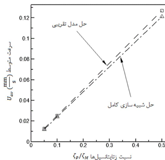
شکل 17 سرعت متوسط محاسبه شده توسط مدل تقریبی H-S (منحنی خط چین) و شبیه‌سازی کامل (منحنی خط - نقطه چین) درون ریزمجرای ناهمگن با الگوی بار (np-np) برای سه مقدار مختلف \zeta_p/\zeta_M
