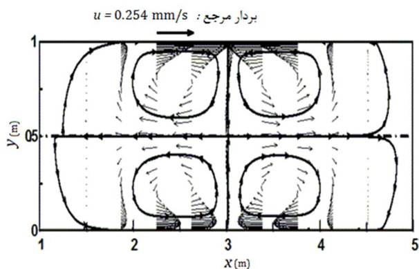
شکل 11 خطوط جریان و بردارهای سرعت در ریزمجرای ناهمگن با الگوی بار (np-np) در قسمت میانی ( 2 < x < 4 ) با استفاده از حل عددی مدل H-S (نیمه بالایی شکل) و حل عددی معادلات ارنست-پلانک (نیمه پایینی شکل)
