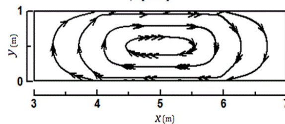
ج) pp-nn
