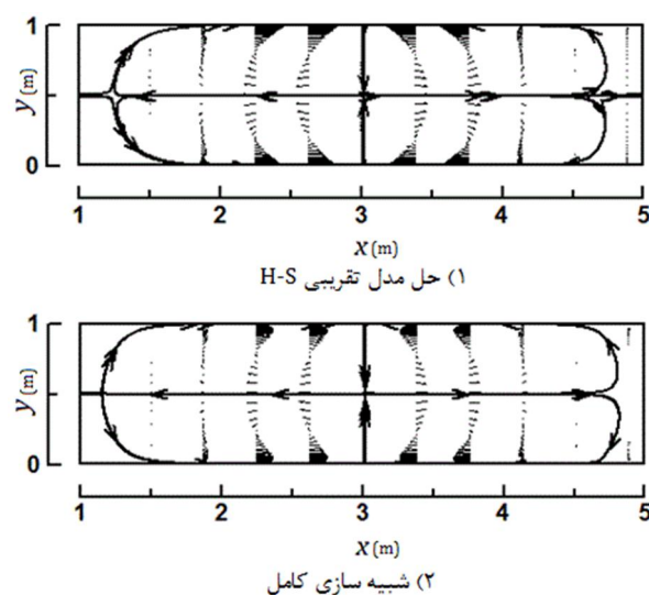
شکل 8 خطوط جریان و بردارهای سرعت در ریزمجرای ناهمگن با الگوی بار (np-np) در قسمت میانی: (1) حل عددی بر مبنای مدل H-S، و (2) حل عددی معادلات ارنست-پلانک
