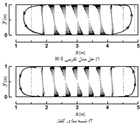
شکل 10 خطوط جریان و بردارهای سرعت در ریزمجرای ناهمگن با الگوی بار (pp-nn) در قسمت میانی: (1) حل عددی بر مبنای مدل H-S، و (2) حل عددی معادلات ارنست-پلانک
