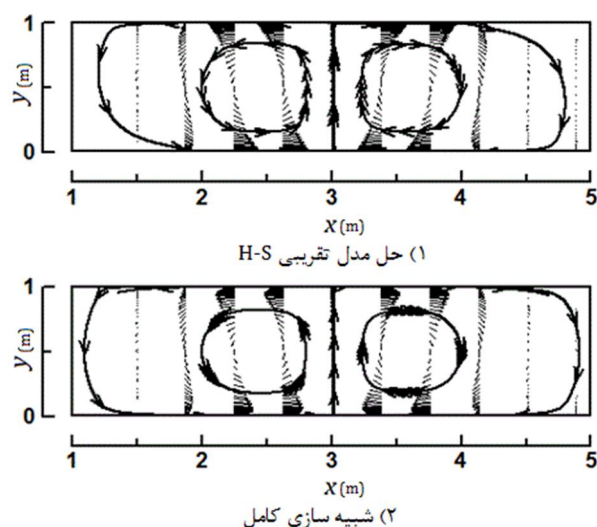
شکل 9 خطوط جریان و بردارهای سرعت در ریزمجرای ناهمگن با الگوی بار (pn-np) در قسمت میانی: (1) حل عددی بر مبنای مدل H-S، و (2) حل عددی معادلات ارنست-پلانک
