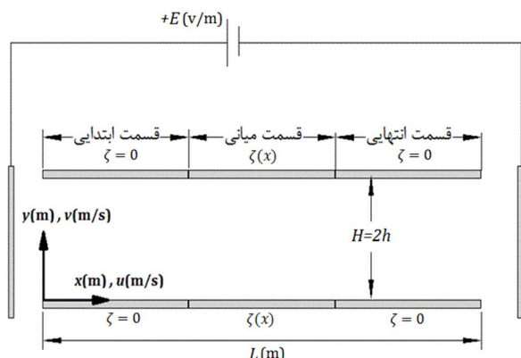
شکل 5 مشخصات ریزمجرای ناهمگن مورد بررسی و محورهای مختصات
